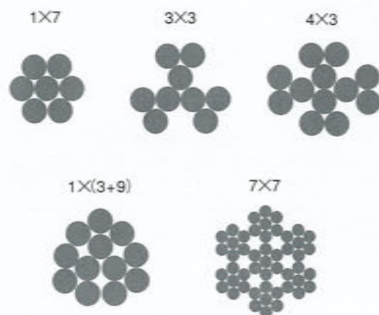
ワイヤー構成 / DIAGRAM / 鋼絲繩構造
