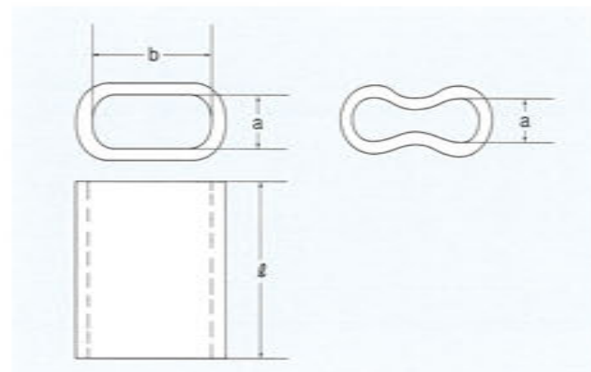
銅ロック/COPPER LOCK/扣環
